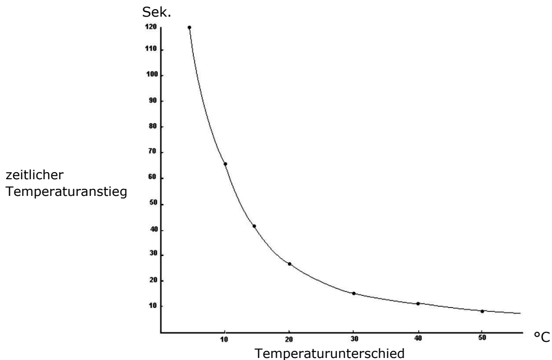
Diagramm für den Temperatur Anstieg/Abfall in Sek.
